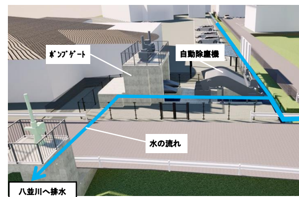
田熊雨水ポンプ場（整備イメージ）
