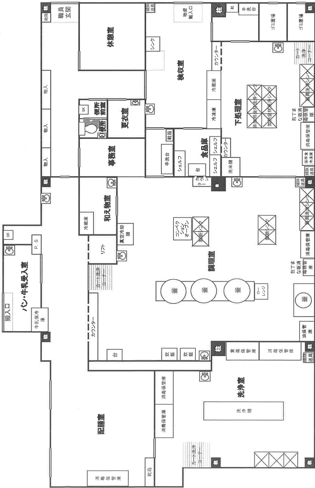
玄海小学校給食室 略図
