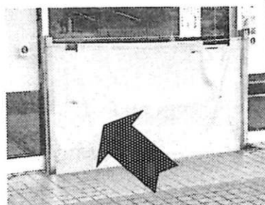
店舗の入口に支柱を立て、シートを設置することで、浸水被害を軽減。
