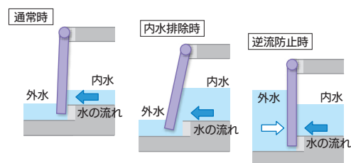
フラップゲートのしくみ
