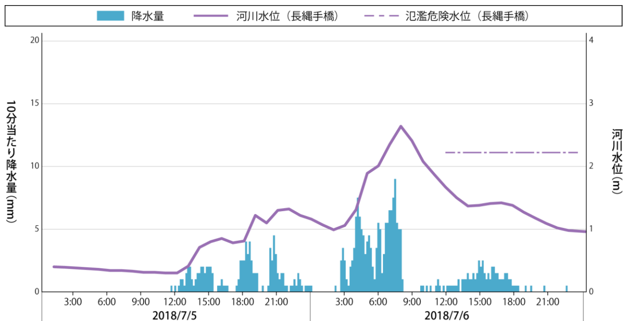
図2-20 降水量および河川水位（長縄手橋）
