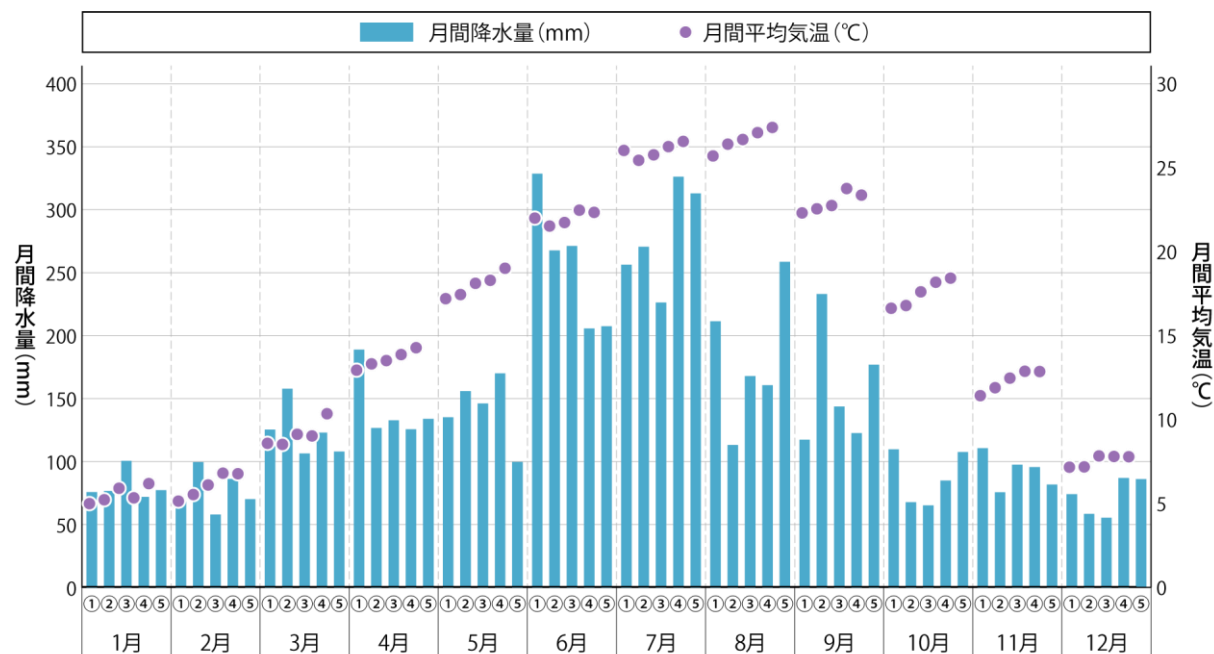
図1-5 年代別の平均気温と降水量の推移
