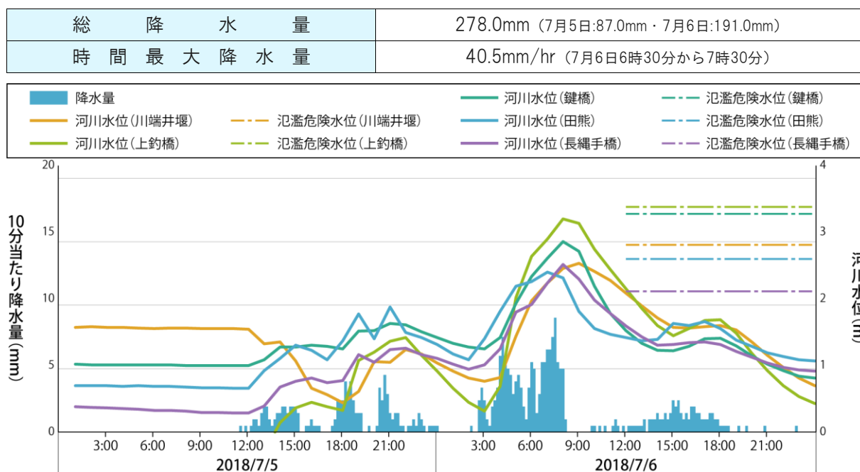
図1-18 降水量と河川水位の推移（平成30年7月豪雨）
