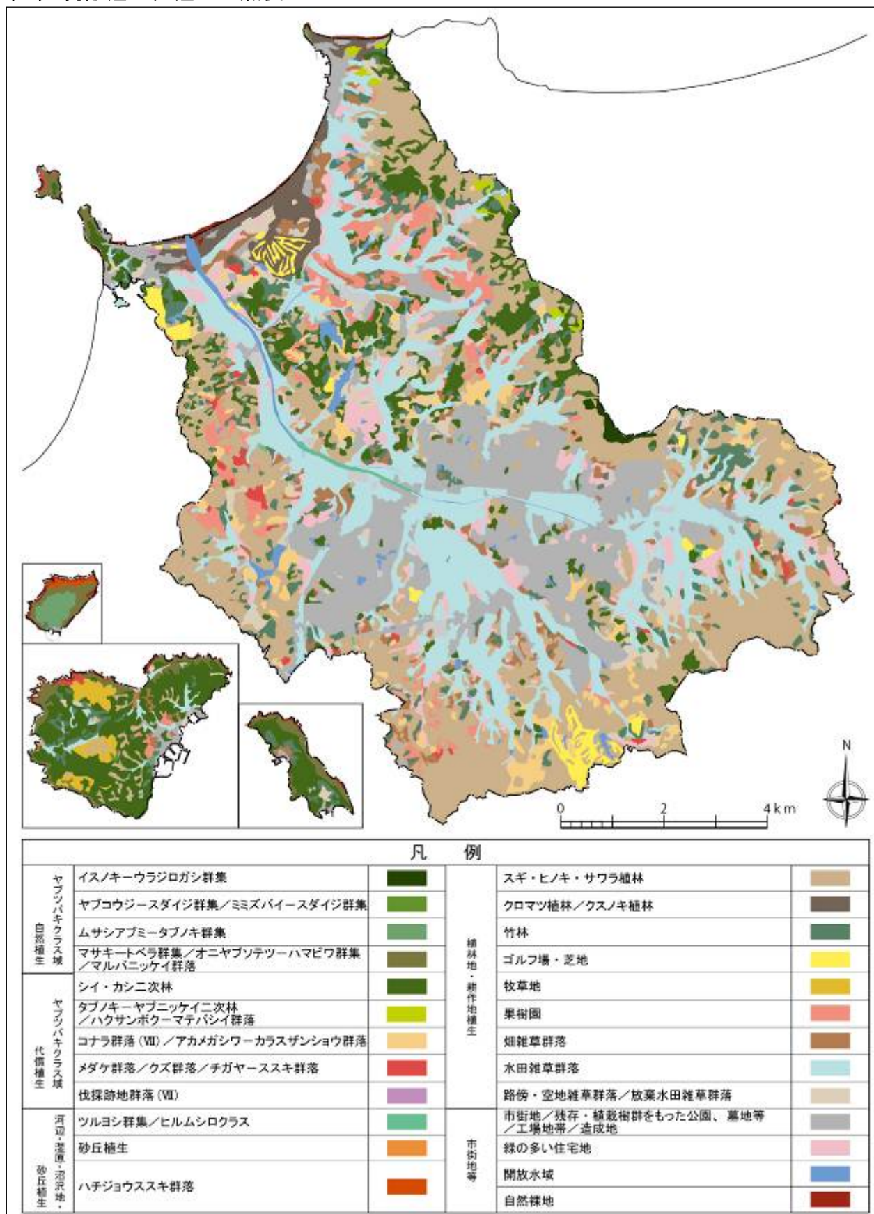
図 植生自然度（自然度の高いものを抜粋表示） [資料：環境省第6回自然環境保全基礎調査（H11～16）]
