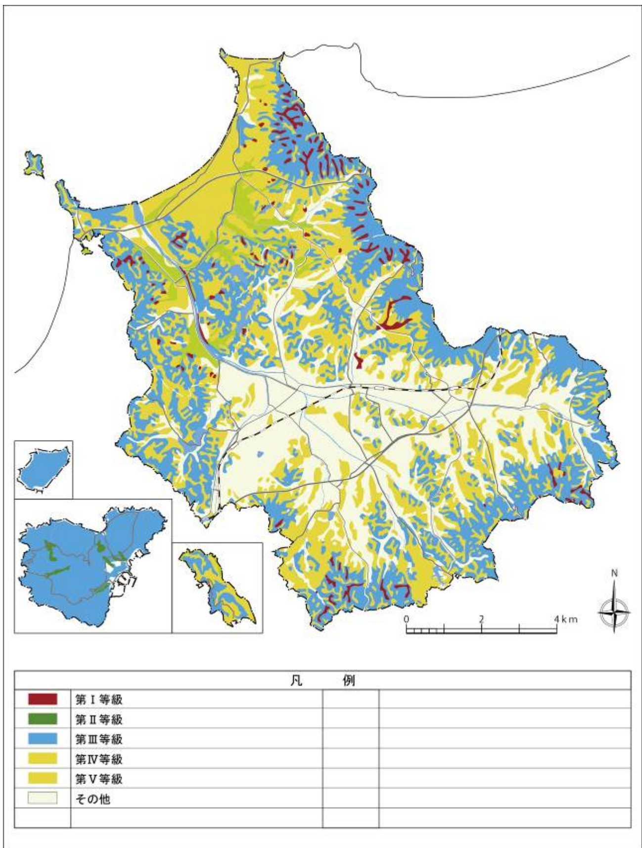
図 土壤生産力図（林地） 〔資料：福岡県土地分類基本調査（S48）（S57）〕
