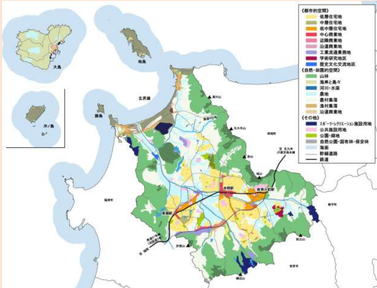
【土地利用方針図】
