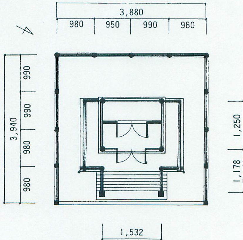
平山天満宮本殿平面図
