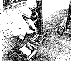
超音波探傷機による検査の事例であり掘削せずに鋼製支柱埋設部の劣化調査が可能となる
