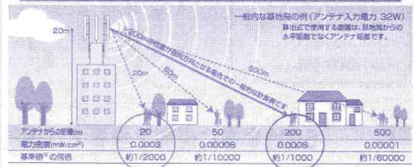
デジタル携帯電話基地局のアンテナから発射される電波の地上での電力密度の例
